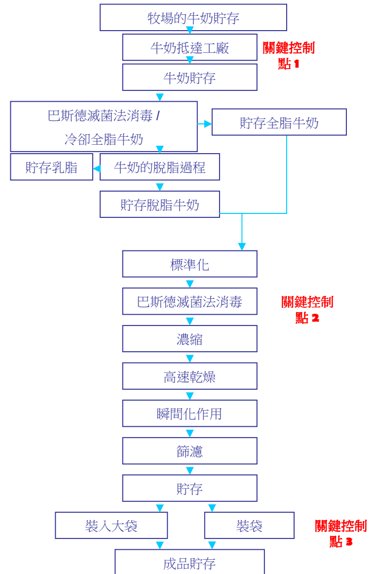
奶粉生產流程圖
